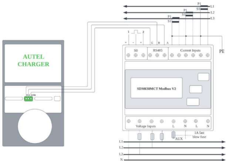
Figure 2-9 Câblage du câble RS485 du compteur d'énergie SDM630MCT-Modbus V2
