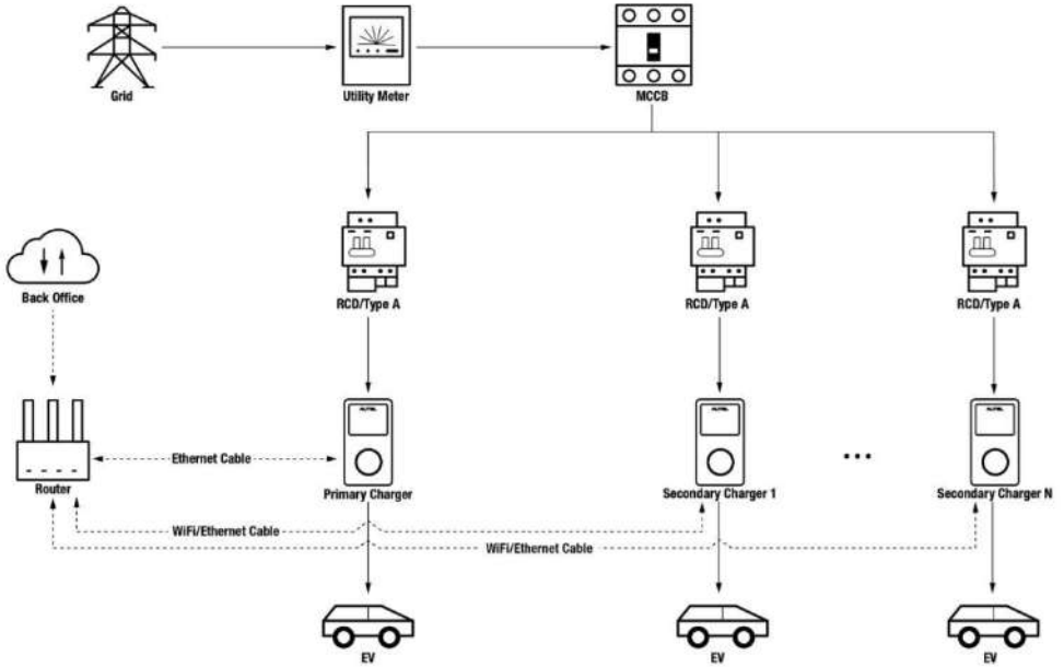
Figure 2-1 Schéma du système (mode DLB)
