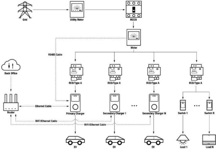
Figure 2-2 Schéma du système (mode ALM)
