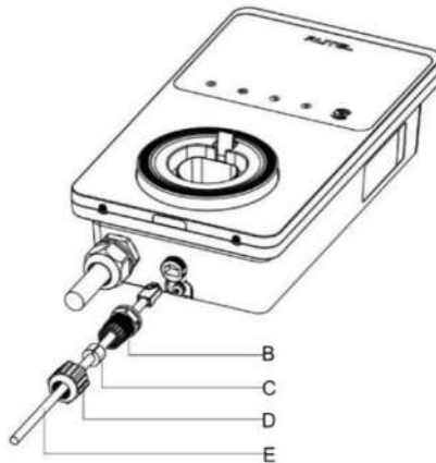
Figure 2-5 Installation du presse-étoupe étanche du câble Ethernet
