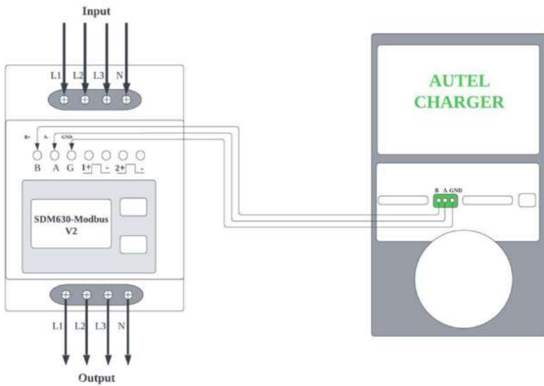
Figure 2-8 Câblage du câble RS485 du compteur d'énergie SDM630-Modbus V2
