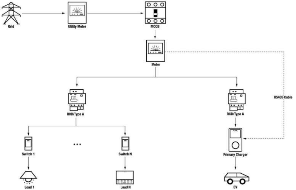
Figure 2-3 Schéma du système (mode ALM)
