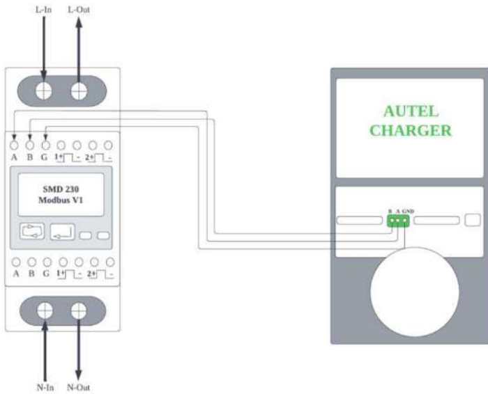
Figure 2-7 Câblage du câble RS485 du compteur d'énergie SDM230-Modbus V1
