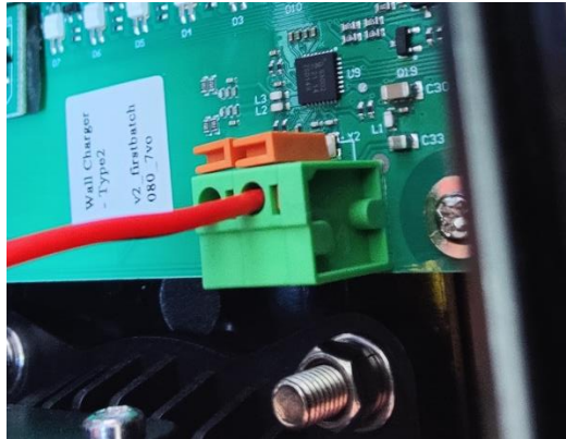
Figure 1 – Connexion de la pince à l'aide des connecteurs à ressort
